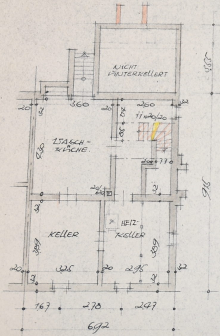
KELLERGESCHOSS.
